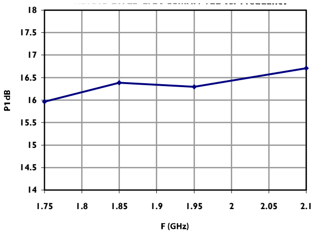
P1dB
