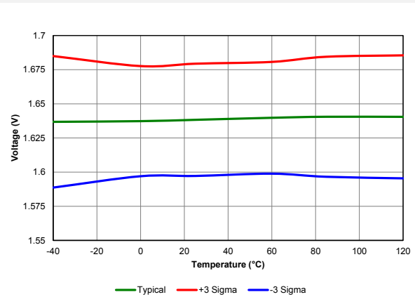
Figure 39-79. POR Release Voltage
