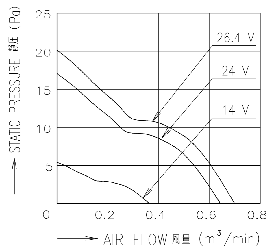
風量-静圧特性例
