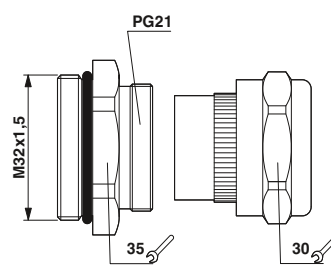
VC-M-KV-PG21/M32 ST / VC-M-KV-PG21...
