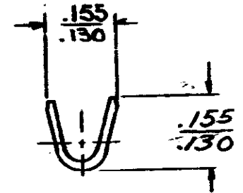
SECT A-A
