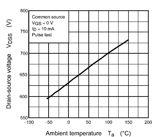
Fig. 8.5 V_{DS} - T_a
