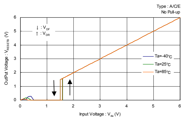
XC6129C ( V_{DF(T)}=1.5V )
