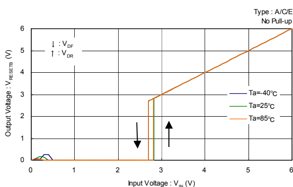
XC6129C ( V_{DF(T)}=2.7V )
