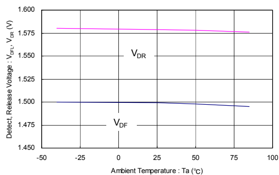
XC6129 ( V_{DF(T)}=1.5V )
