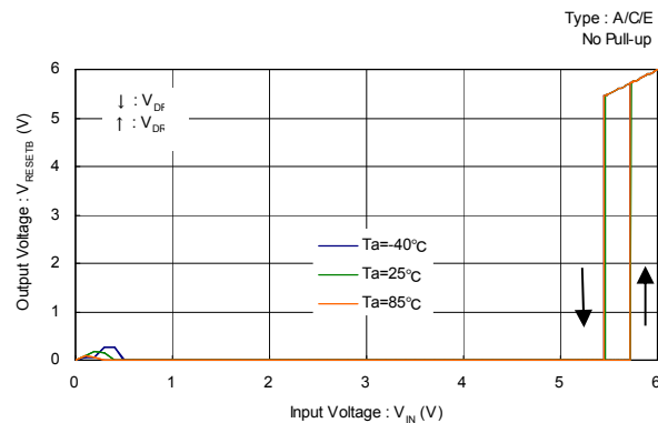
XC6129C ( V_{DF(T)}=5.5V )
