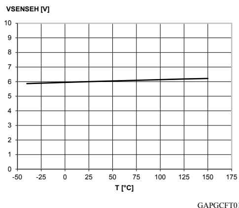
Figure 34. V_{senseh} vs. T_{case}
