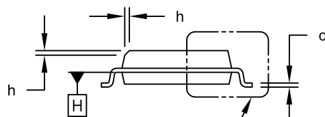
VIEW A-A
