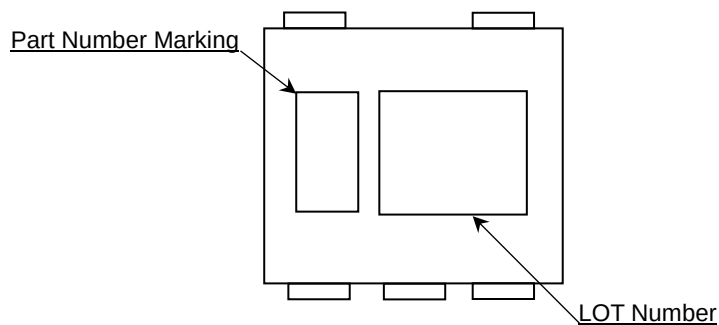
SSOP5(TOP VIEW)
