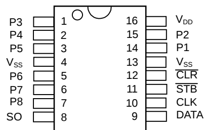
NJU3712AV
