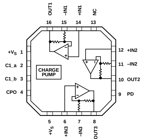
ADA4859-3
