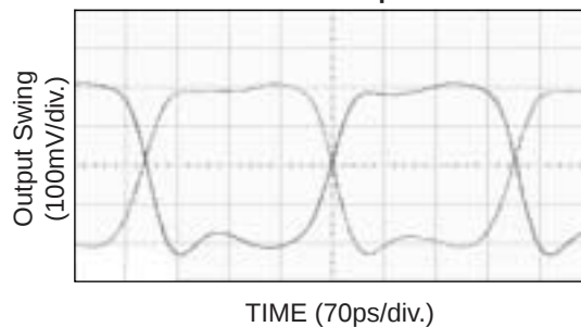
2GHz Output
