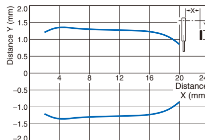
Reflective E32-L56E□
