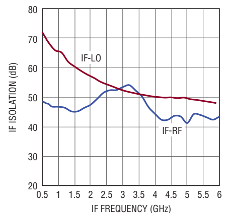
IF Isolation
