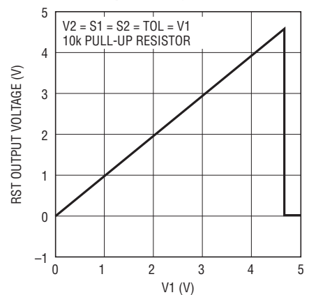
\text{RST} Output Voltage vs V1
