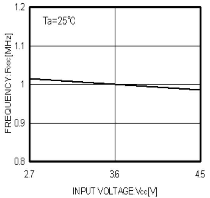
Fig.79 V CC -F osc
