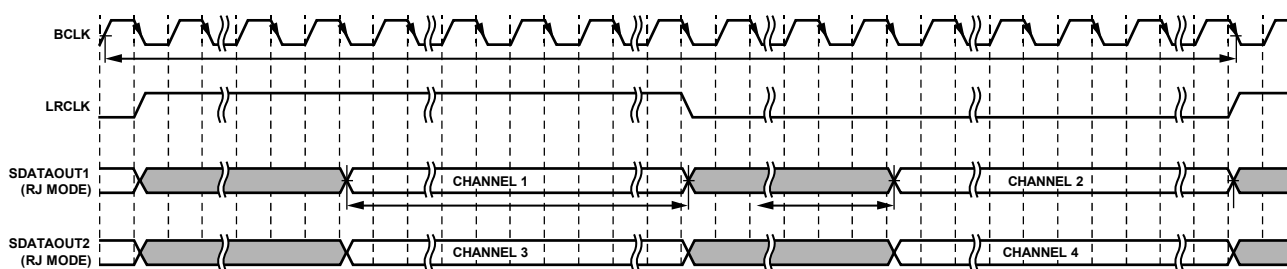
Figure 25. LJ Audio Format
