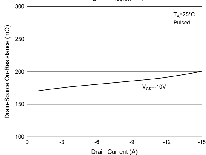
Fig. 6 - R_{DS(ON)} — I_D
