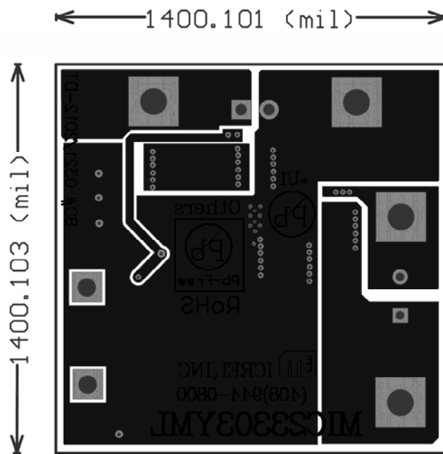
Bottom Layer
