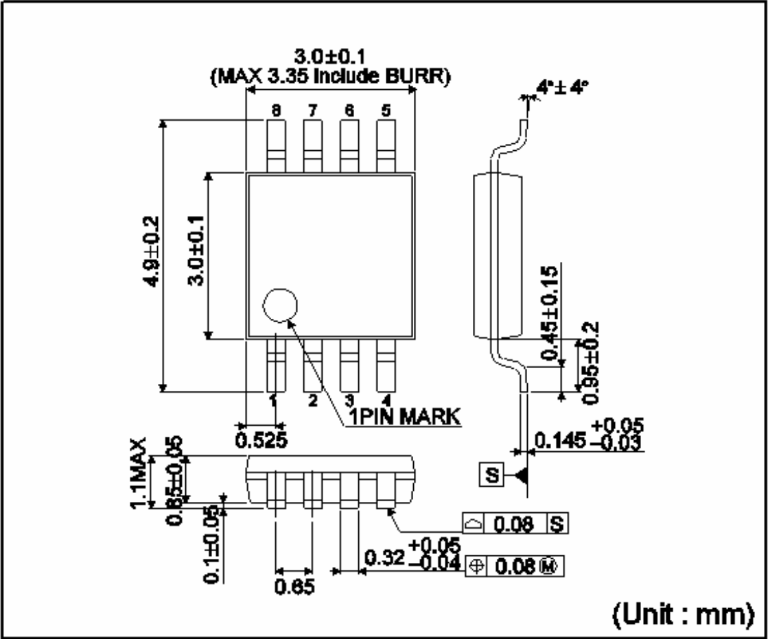
TSSOP-B8J
