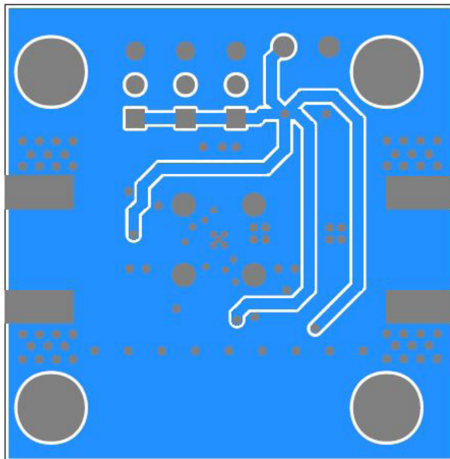
MAX2248 EV Kit—Gerber Bottom
