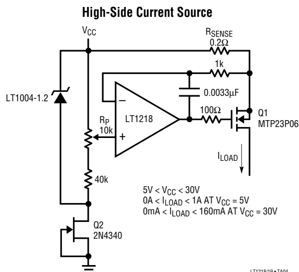
LT1218/19 • TA04
