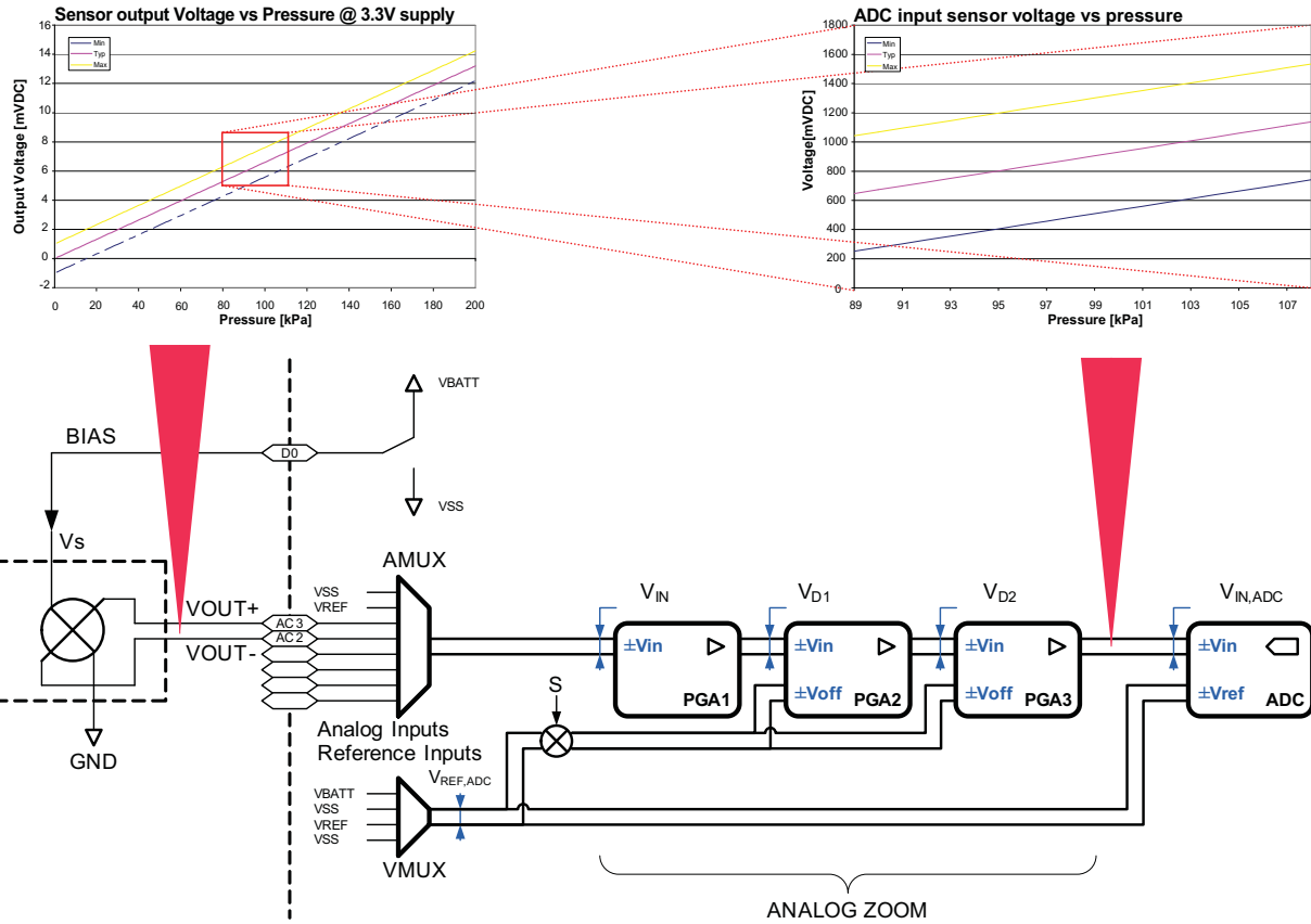
Figure 42. PGA Parameters
