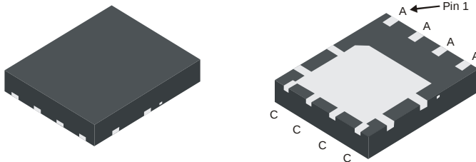
POWERDI5060-8
