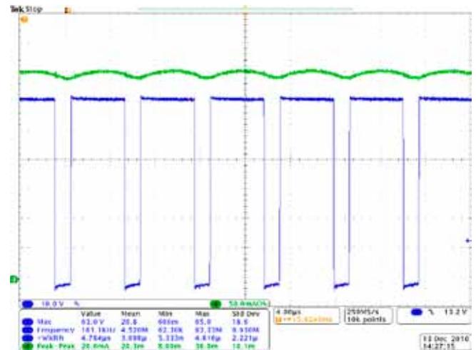
Fig.4: 60V Input
