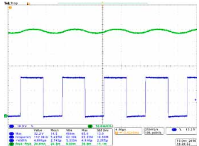
Fig.2: 30V Input
