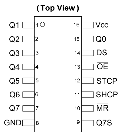
SO-16 / TSSOP-16
