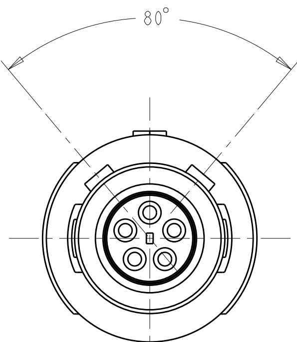
80° KEYING SCALE 4:1
