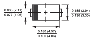
DO-214AA
