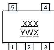
SOT25 / SOT353
