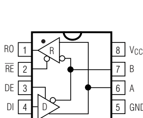
DIP/SO
