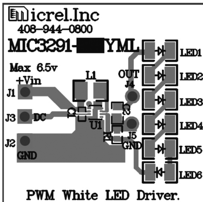
Top Layer
