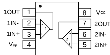
SO-8/MSOP-8
