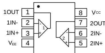
SO-8/MSOP-8
