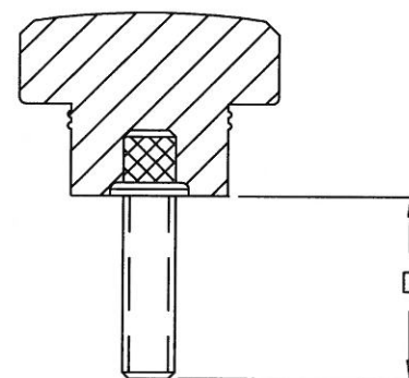
THREADED STUD
