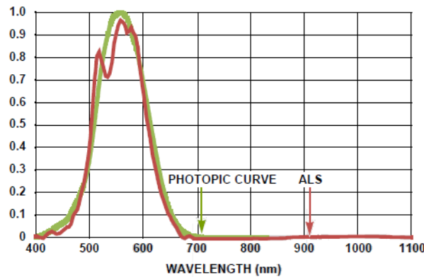
Figure 9 ALS Sensitivity vs Wavelength
