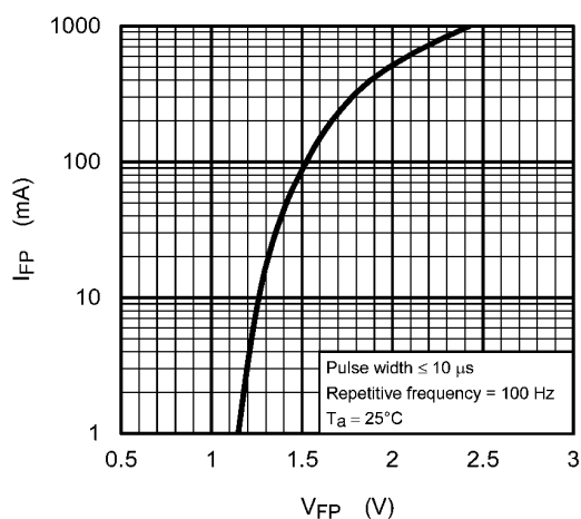
Fig. 12.5 I_{FP} - V_{FP}
