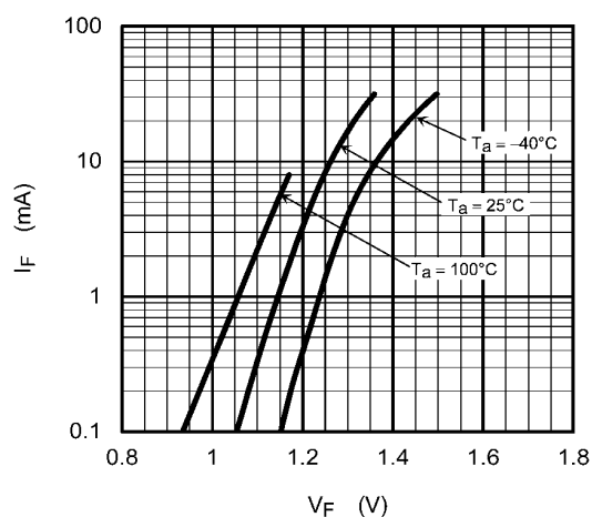
Fig. 12.3 I_F - V_F
