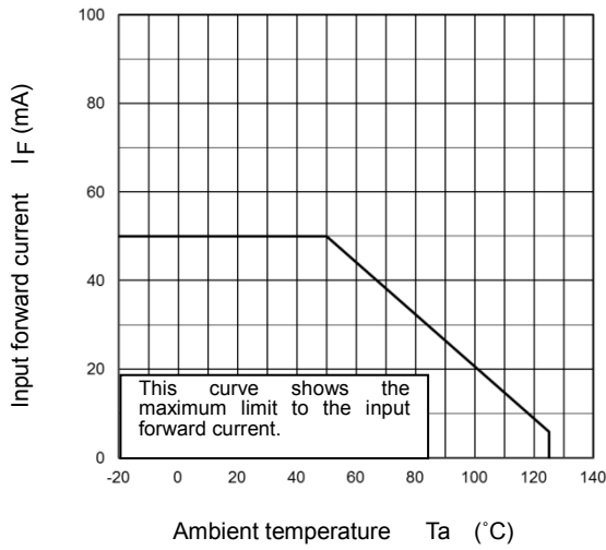
I_F - T_a
