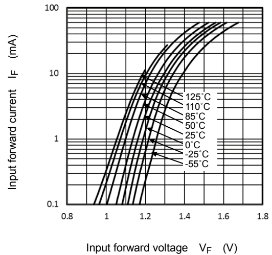
I_{FP} - V_{FP}
