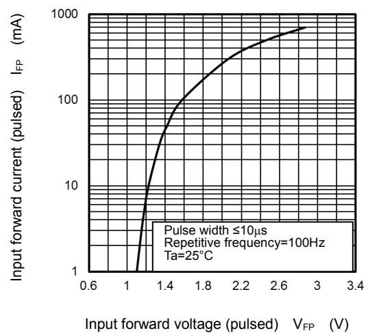
I_{FP} - V_{FP}
