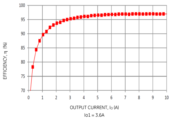
Fig 9a: Efficiency
