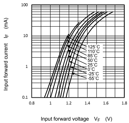
I_{FP} - V_{FP}
