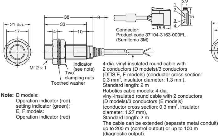
Fig. 8 : E2E-X3D□-N E2E-X2E□/F□
